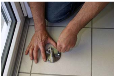
Stellfüße mit beigefügten Dübeln und Schrauben befestigen
