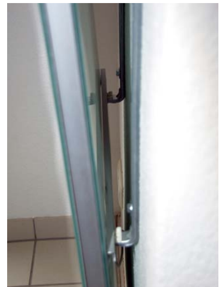
Glasheizkörper in die unteren Aufhängevorrichtungen der Wandhalterungen einhängen
